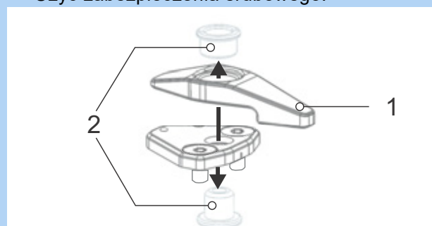
Rysunek 82: Połączyć dźwignię zabezpieczającą z płytą podstawy
