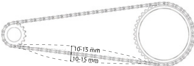
Rysunek 188: Kontrola naprężenia łańcucha
