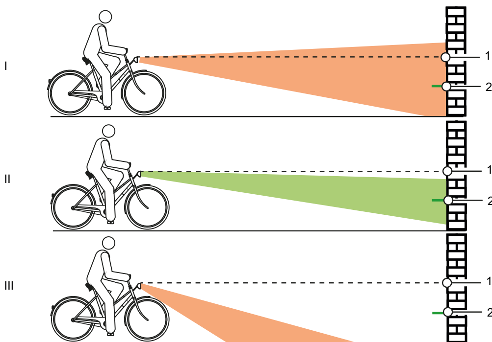
Rysunek 129: Światło ustawione za wysoko (1), prawidłowo (2) i za nisko (3)
