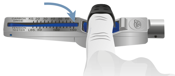
Rysunek 180: Palec wskazujący na przyrządzie pomiarowym
