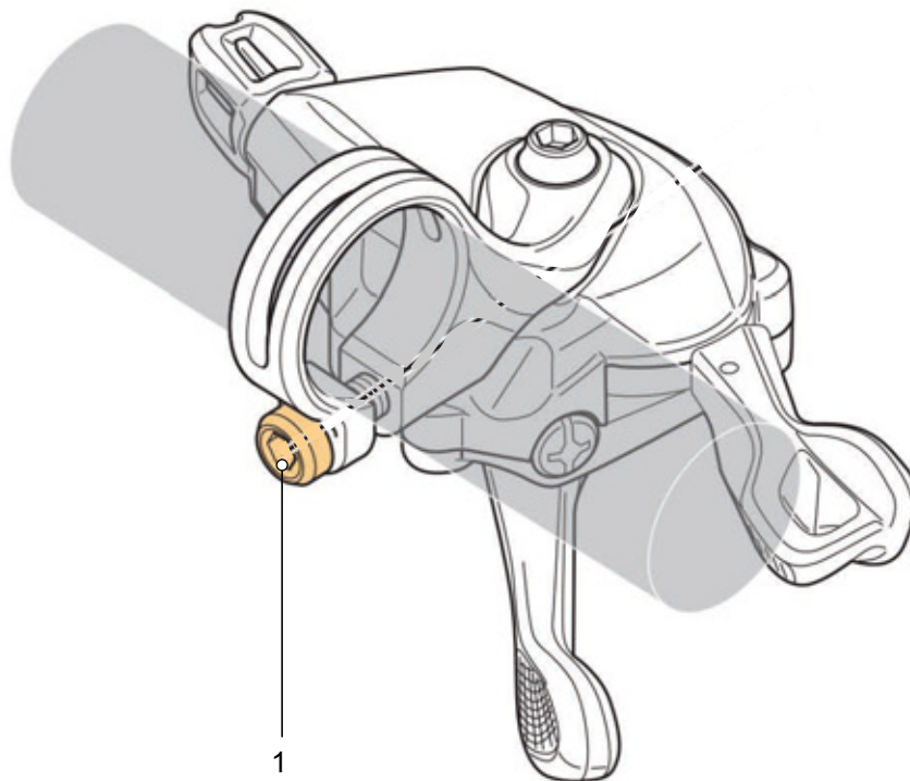
Rysunek 122: Położenie śruby mocującej dźwignię przerzutki SHIMANO (1)
