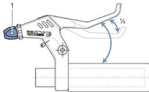
Rysunek 165: Obracać śrubę regulacyjną (1), aż hamulce zatrzasną się po 1/3 skoku hamulca ręcznego
