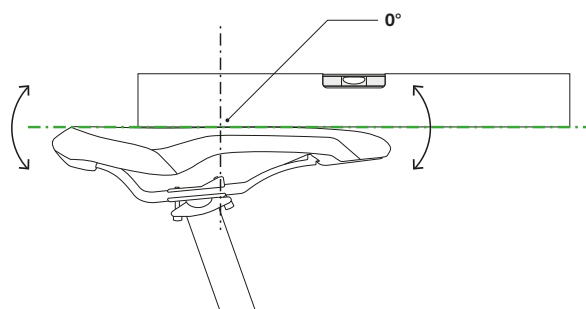
Rysunek 106: Poziome ustawienie siodełka z nachyleniem 0° jego środkowej części
