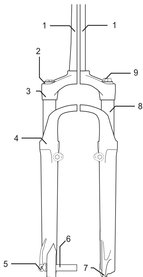
Rysunek 14: Przykładowy stalowy widelec amortyzowany SR SUNTOUR
