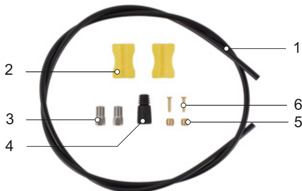
Rysunek 26: Elementy przewodu hamulcowego
