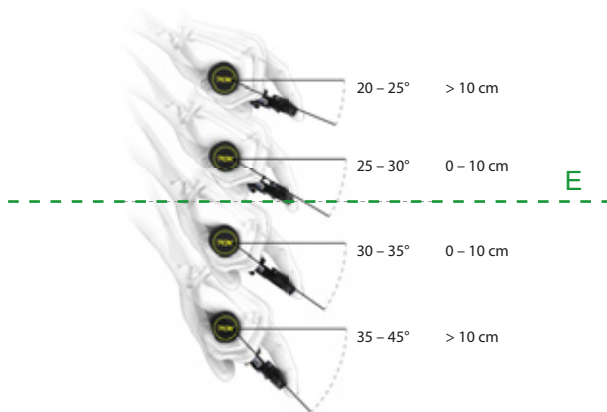
Rysunek 120: Kąt nachylenia hamulca
