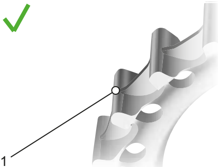
Rysunek 177: Optymalny profil zębów
