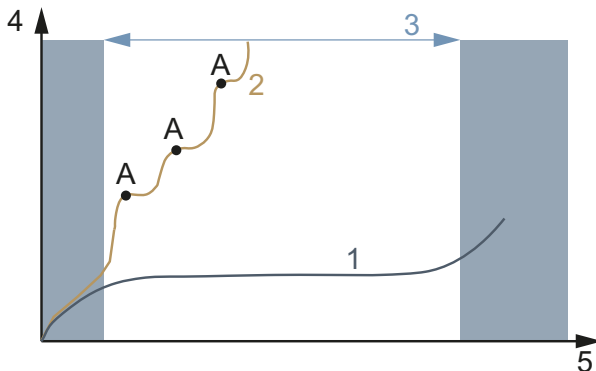
Rysunek 158: Wykres zużycia, czas eksploatacji (x) w stosunku do zużycia materiału (y)
