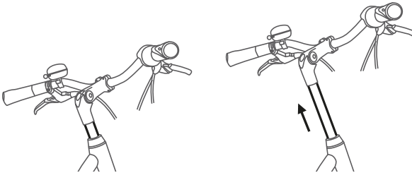
Rysunek 111: Regulacja wysokości mostka wpuszczanego
