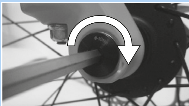
Rysunek 66: Dokręcić oś zgodnie z kierunkiem strzałki.
