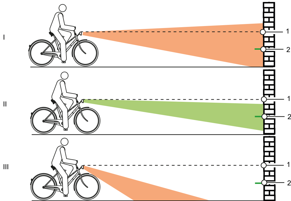
Rysunek 187: Światło ustawione za wysoko (1), prawidłowo (2) i za nisko (3)
