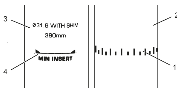
Rysunek 103: Widok szczegółowy sztyc podsiodłowych, przykłady oznaczenia minimalnej głębokości osadzenia
