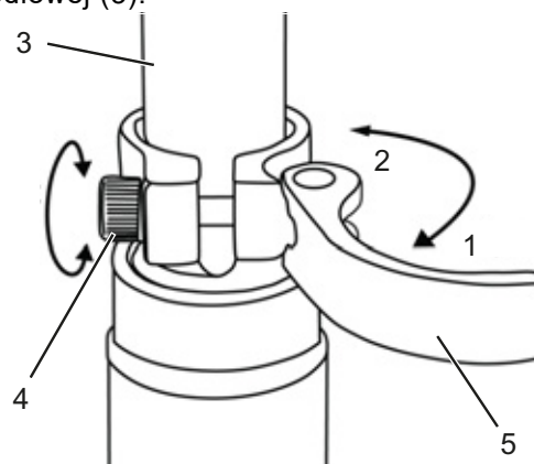
Rysunek 102: Zacisk szybkomocujący sztycy podsiodłowej w pozycji otwartej
