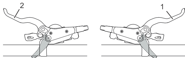
Rysunek 149: Ręczny hamulec tylny (1) i przedni (2), przykład – hamulec SHIMANO
