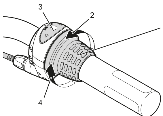
Rysunek 154: Przykładowy mechanizm zmiany przerutek marki SHIMANO Nexus
