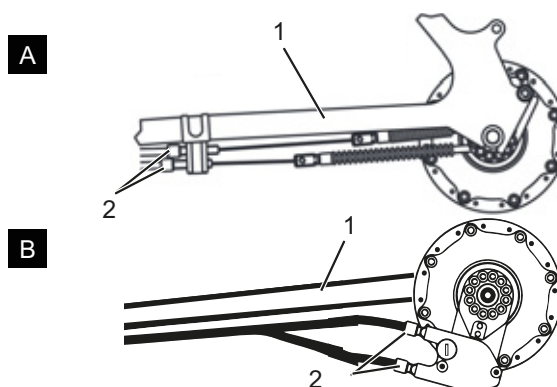
Rysunek 191: Nakrętki regulacyjne (2) w dwóch alternatywnych wersjach (A i B) dwucięgnowego mechanizmu przerzutki na rurze dolnej tylnego trójkąta (1)
