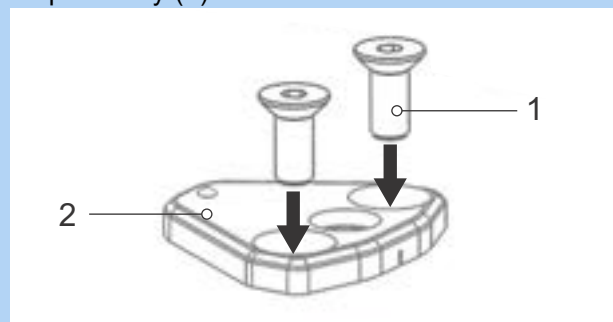
Rysunek 81: Wkładanie śrub z łbem stożkowym w płytkę podstawy
